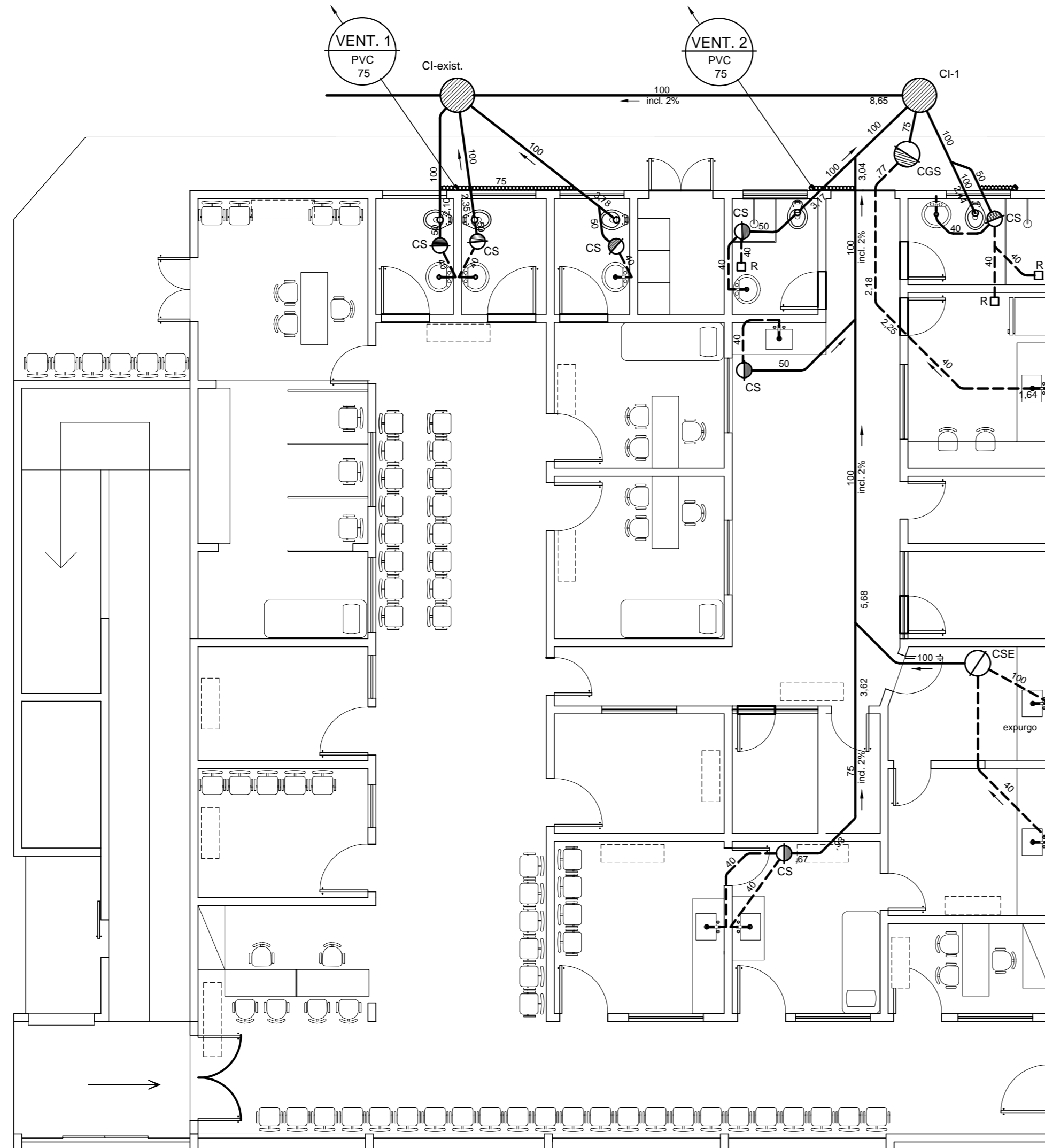
PLANTA BAIXA - TÉRREO ESGOTO 1:75
